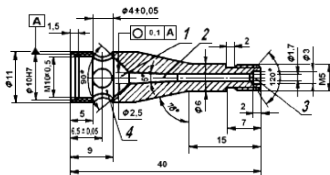
Рисунок Е.4 - Трубка газовой горелки
